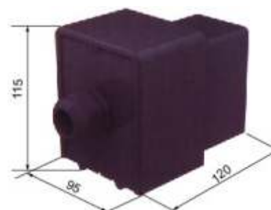
Замыкающий подвод
